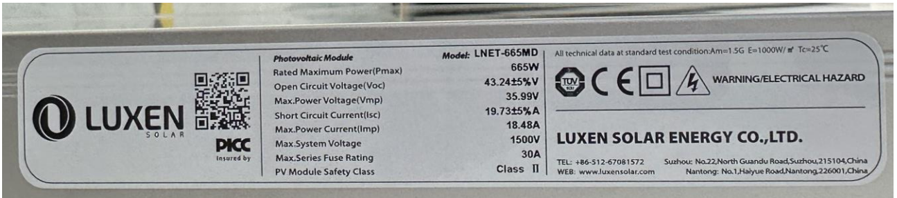
Placa de marcação da Amostra
